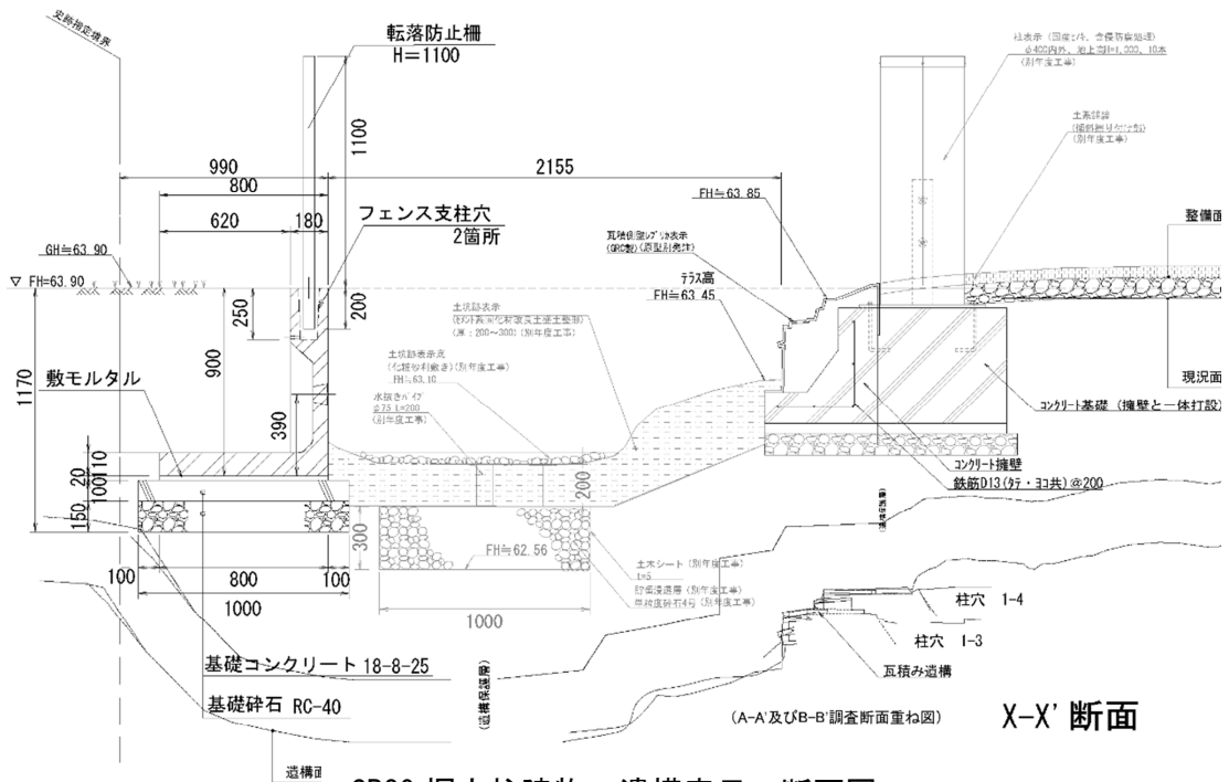
SB39 掘立柱建物 遺構表示 断面図
